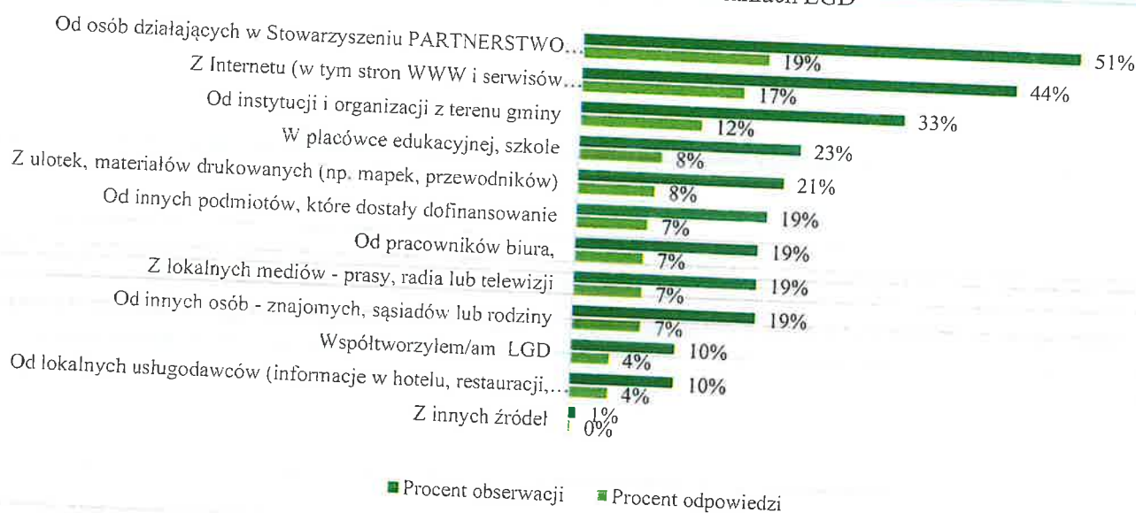
Rysunek 4 Źródła wiedzy beneficjentów o działaniach LGD
