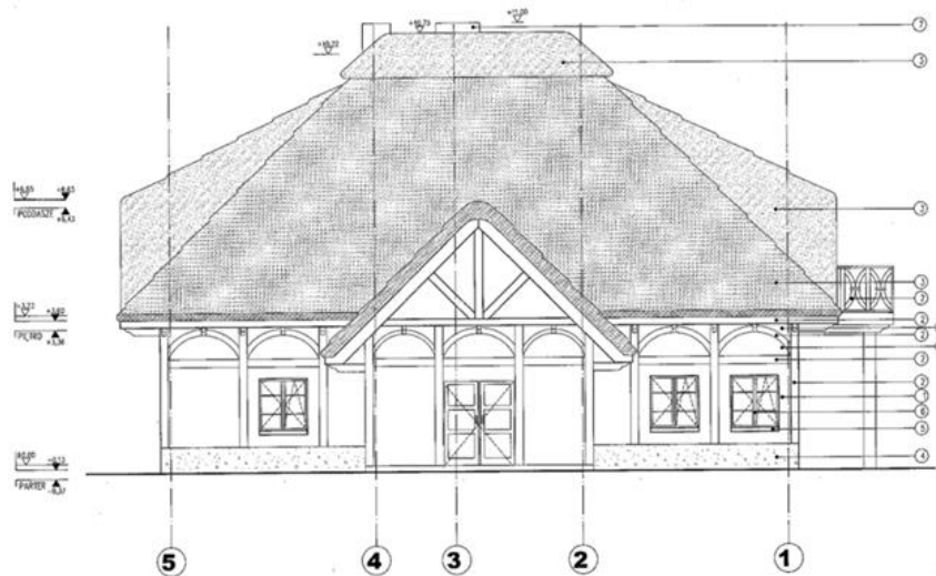
elewacja północno-zachodnia
